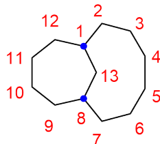
bicyklo[6.4.1]tridekan
