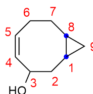
bicyklo[6.1.0]non-4-en-3-ol
