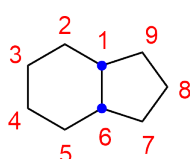
bicyklo[4.3.0]nonan
